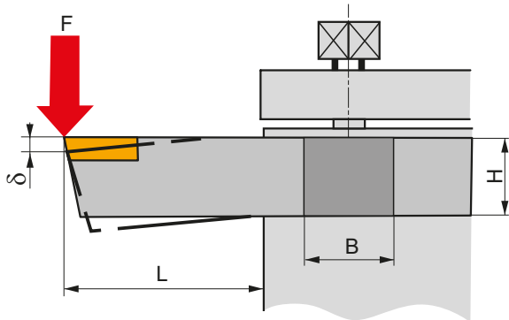
Напряжения при изгибе
