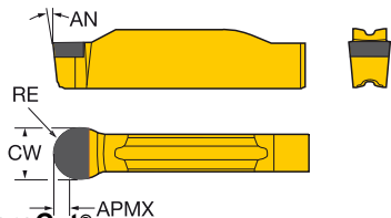
Однолезвийные пластины CoroCut®
