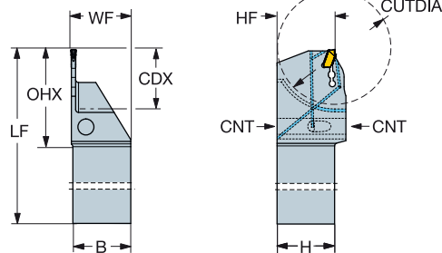
QD-R/LF..C..D
