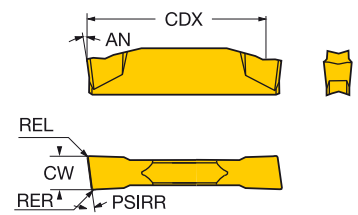
R123x2-CM
