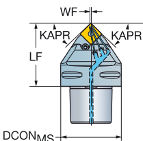
Cx-PSDNN..HP 45.0°
