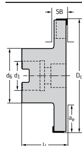
Цилиндрическая Бодринг Quermitnahme DIN 138
