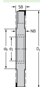
Цилиндрическая Бодринг Längsnut DIN 138
