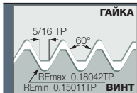
ВИНТ
